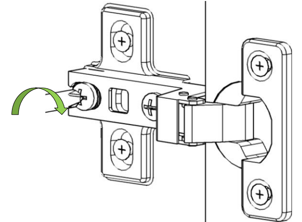
İLERİ GERİ KAPAK AYARI
