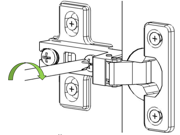
SAĞ - SOL KAPAK AYARI
