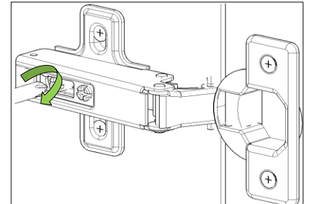
DÜZ MENTEŞE İÇİN İLERİ GERİ KAPAK AYARI
