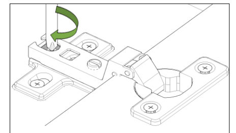
SÜPER DEVE MENTEŞE İÇİN İLERİ - GERİ KAPAK AYARI
