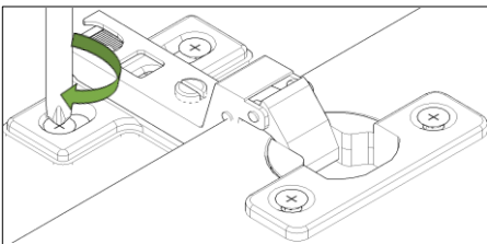
SÜPER DEVE MENTEŞE İÇİN SAĞA - SOLA KAPAK AYARI
