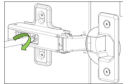
DÜZ MENTEŞE İÇİN SAĞA - SOLA KAPAK AYARI
