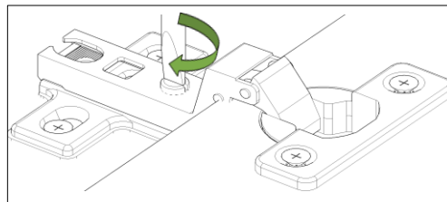
SÜPER DEVE MENTEŞE İÇİN YUKARI - AŞAĞI KAPAK AYARI
