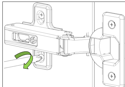
DÜZ MENTEŞE İÇİN YUKARI AŞAĞI KAPAK AYARI
