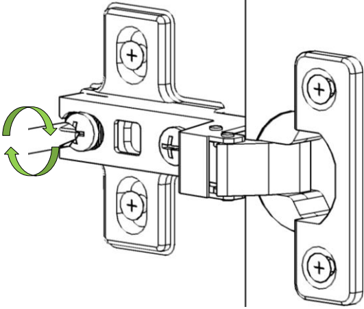
İLERİ GERİ KAPAK AYARI
