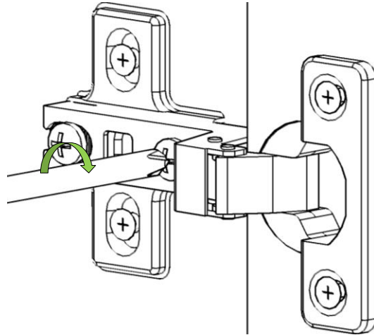
SAĞA - SOLA KAPAK AYARI
