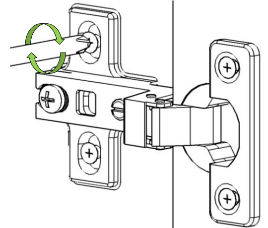
YUKARI AŞAĞI KAPAK AYARI
