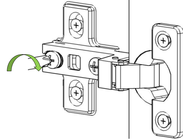
İLERİ GERİ KAPAK AYARI
