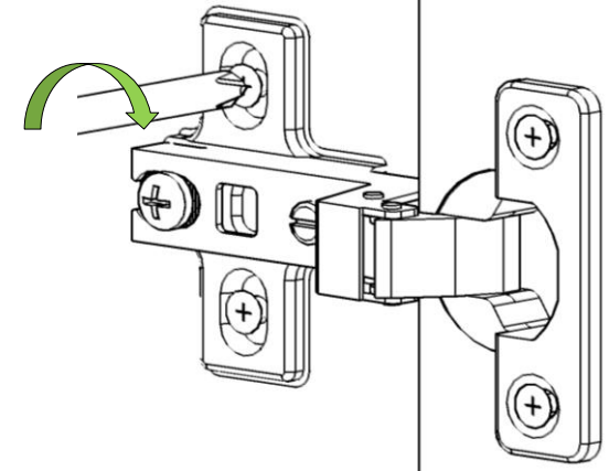
YUKARI AŞAĞI KAPAK AYARI
