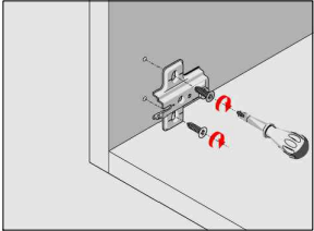
Hinge
