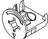
MİNİFİX GÖVDE
